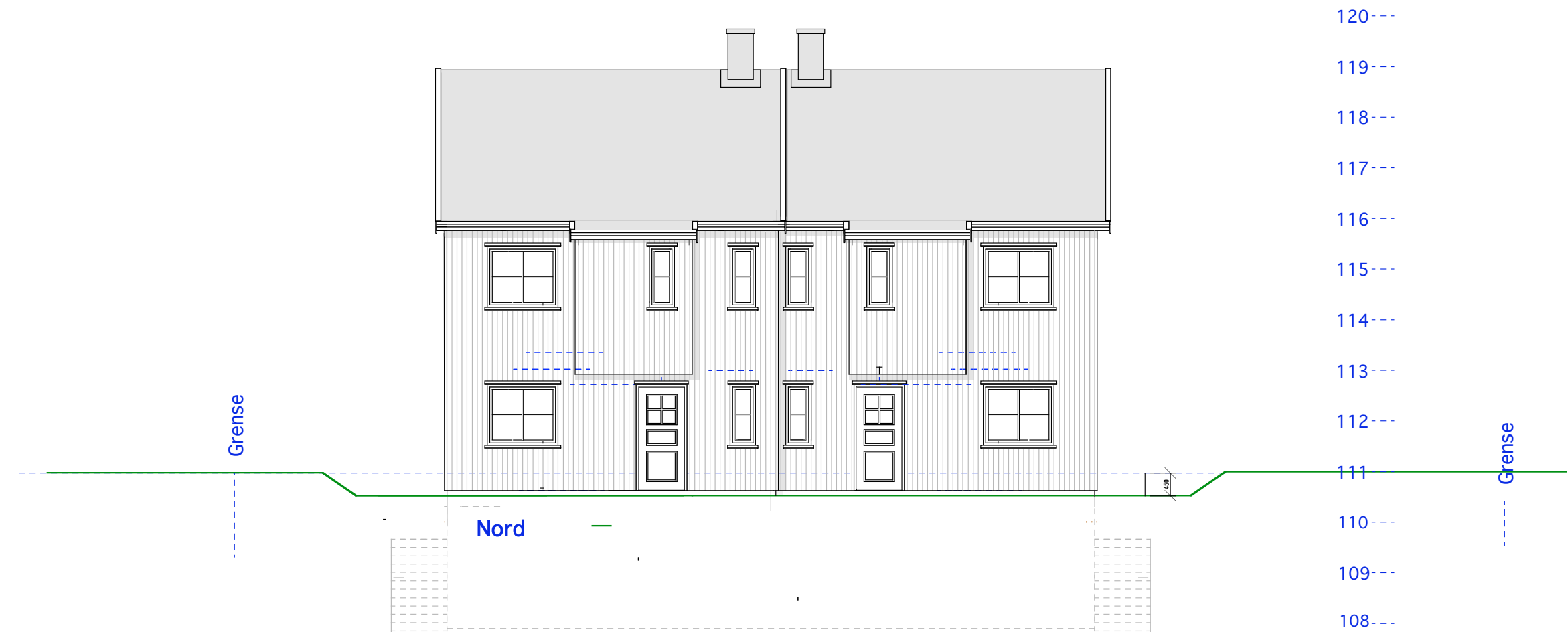
E.1-4 Fasade nord og syd
