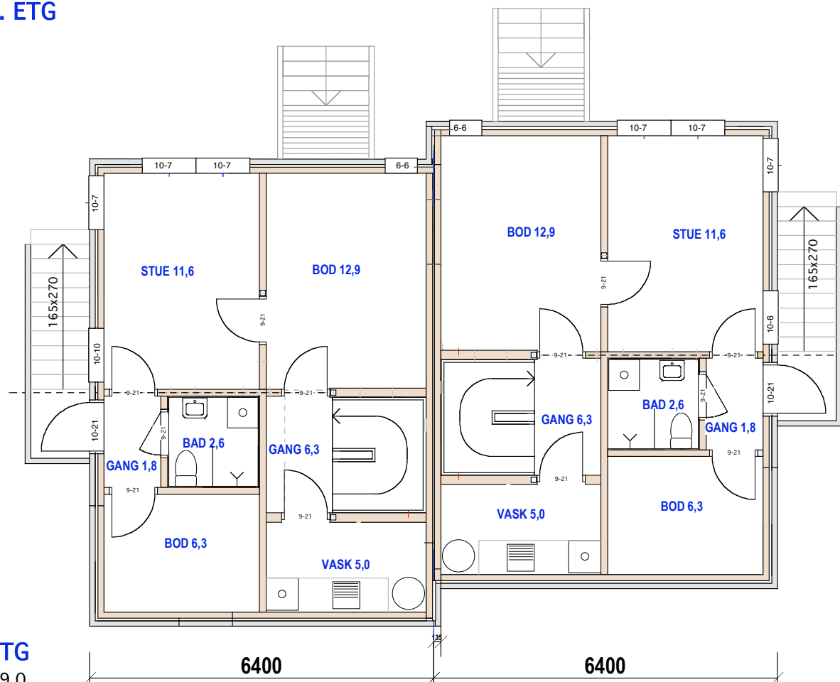
E.1-3 Plan 1. etg og u.etg
